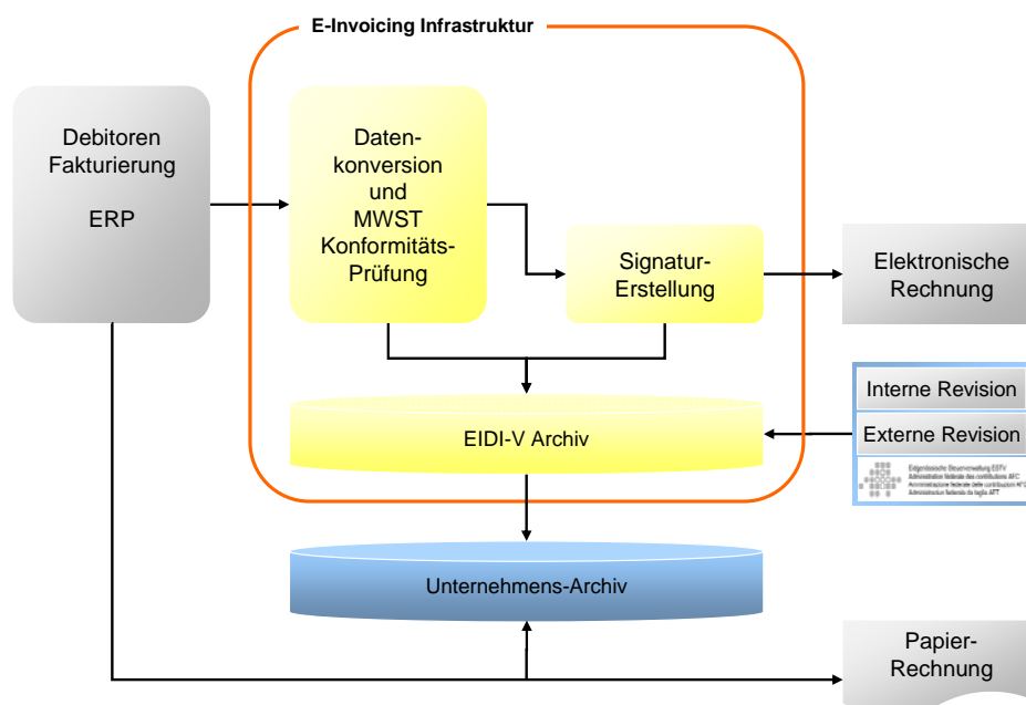
Übersicht E-Invoicing Prozess für Rechnungssteller
